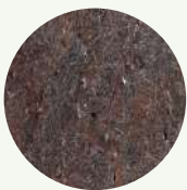
Vesta
